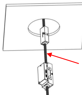
Conduit flexible de fixation QDS
